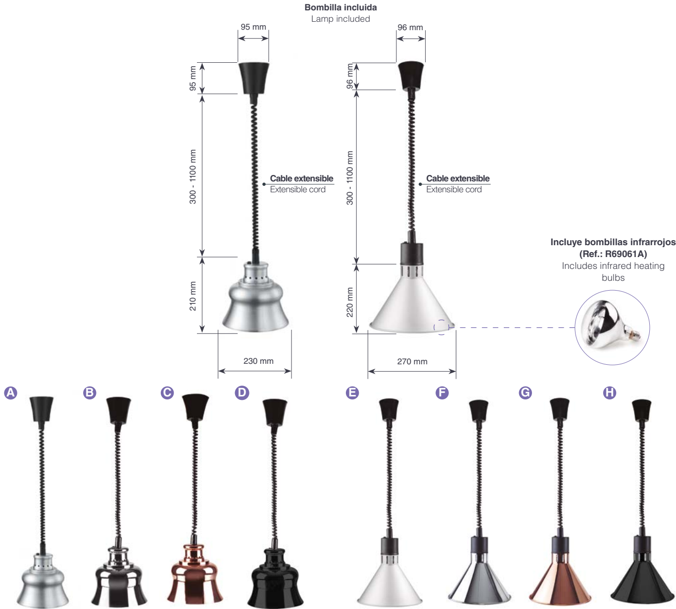
Lámparas de calentamiento extensibles Lampe de chauffage câble extensible · Infrarot Wärmelampe Kabel ausziehbar Infrared heating lamp extensible · Lâmpara calor infravermelho cabo extensível
